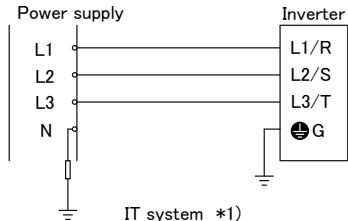
IT system *1)
