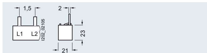
5ST3 705-2HG
