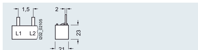
5ST3 710-2HG
