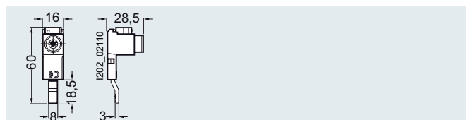
5ST3 770-0HG
