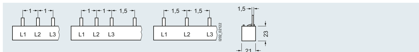
5ST3 710-0HG
