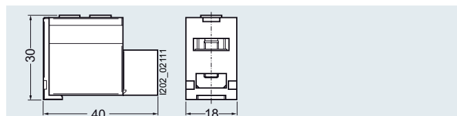
5ST3 770-1HG
